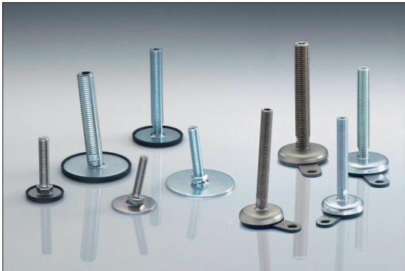
levelling feet GN 440/ GN 440.5
